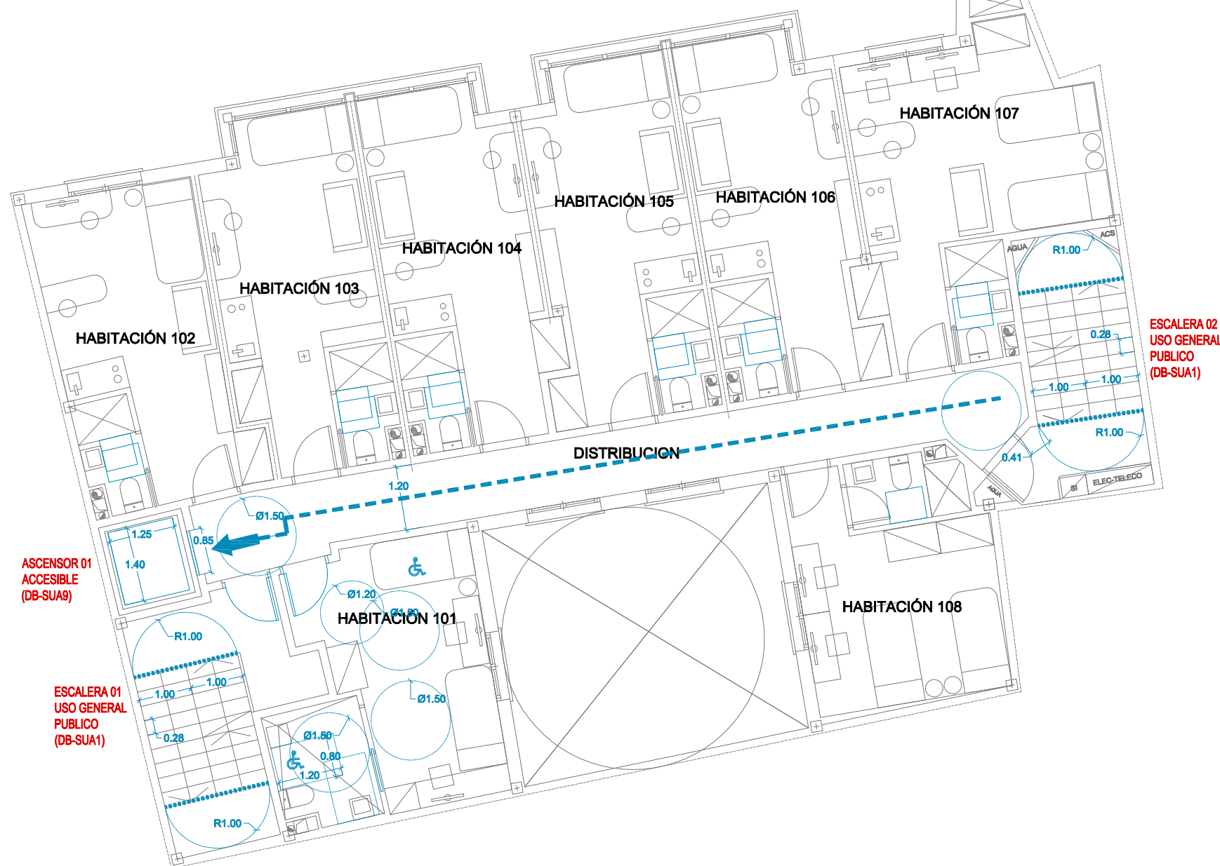
PLANTA PRIMERA
